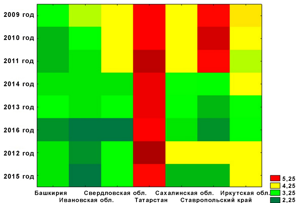
Рис. 2. Двухходовое объединение кластеров заболеваемости среди исследуемых территорий
