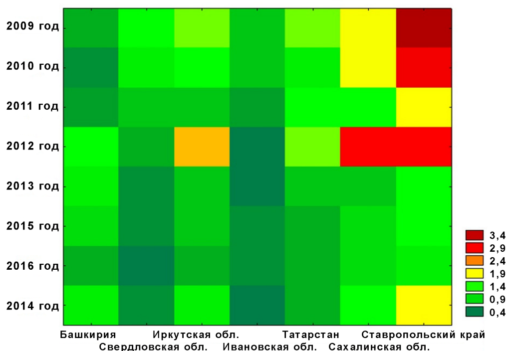
Рис. 3. Двухходовое объединение кластеров смертности от инсульта среди исследуемых территорий
