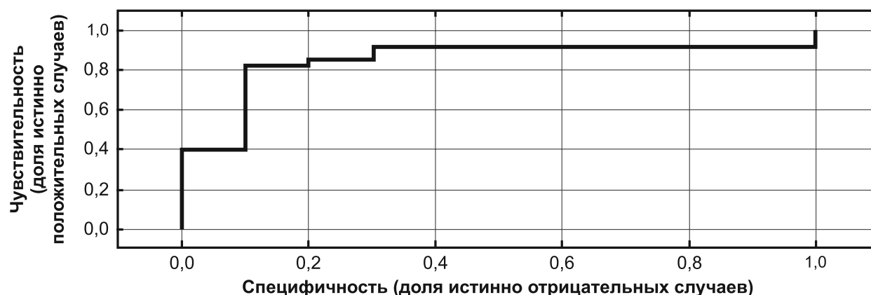
Рис. 1. ROC-кривая для MLP 22-9-2; 100:85:95.
