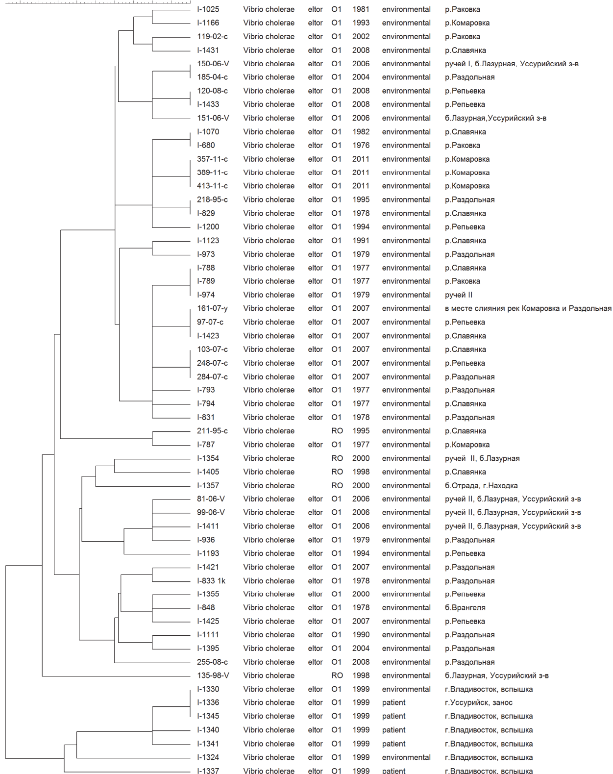
Рис. 1. Дендрограмма, построенная по результатам MLVA-типирования (с использованием алгоритма UPGMA) штаммов V.cholerae , выделенных в период эпидемиологического благополучия и эпидемических осложнений на территории Приморского края.
